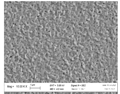
Fig.7: Top view poly layer GaP/Al su Si
