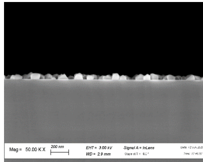
Fig.6: Cross section nucleazione GaP/Al su Si
