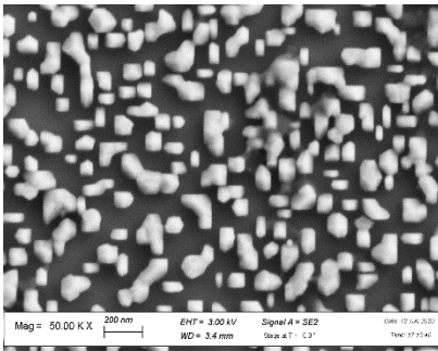
Fig.5: Top view nucleazione GaP/Al su Si
